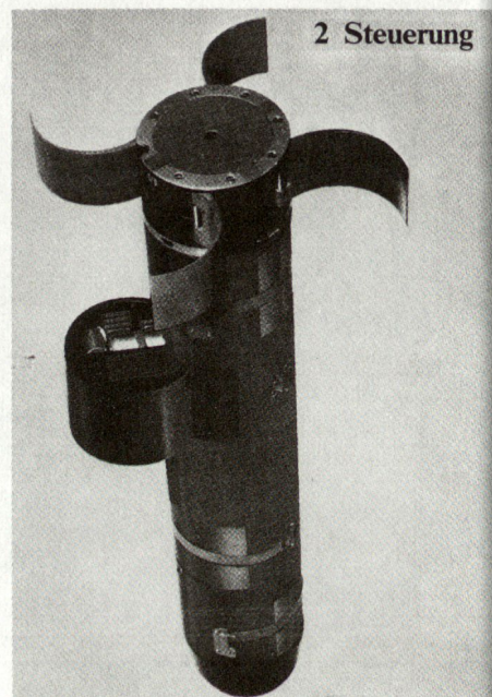
Durch den Infrarotsensor und die Flügelsteuerung wird das Geschoss über ein Panzerziel gebracht.
